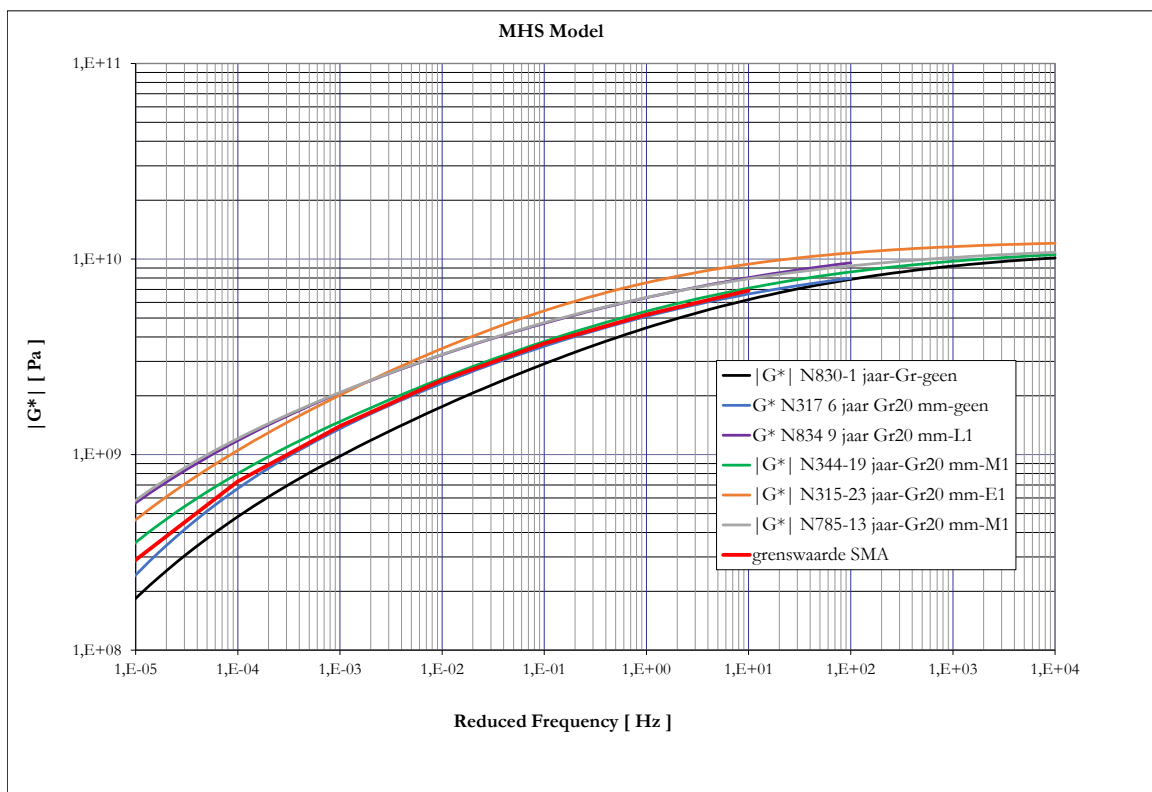
Figuur 7 Mastercurves@-10°C granulormastiek uit bovenste 20 mm van de deklaag
