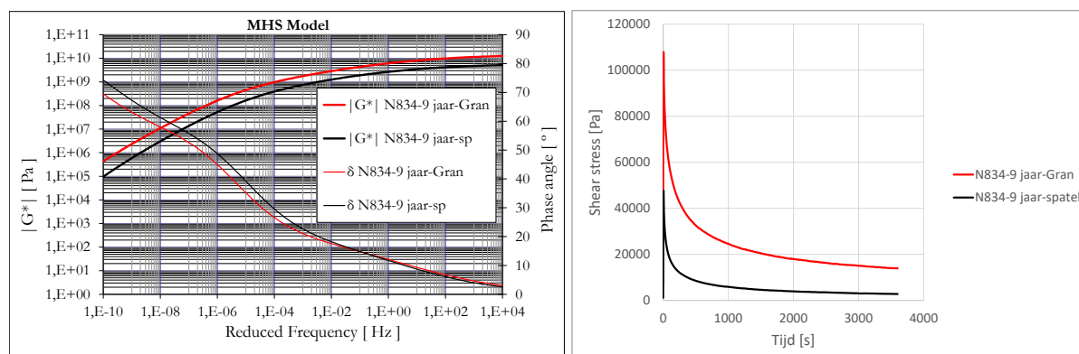
Figuur 5 Mastercurve en relaxatiekromme spatel- en granulatomastiek
