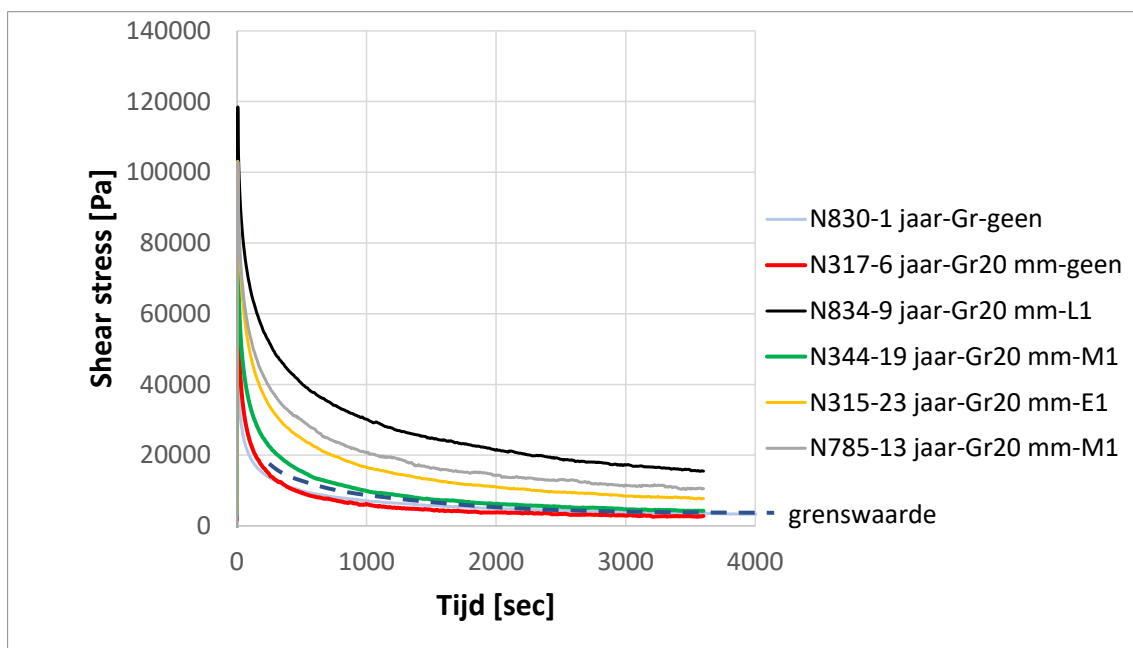
Figuur 9 Relaxatiekrommen granulatormastiek uit bovenste 20 mm van de deklaag
